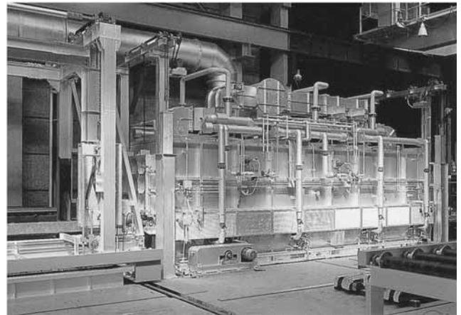
ローラーハース式連続焼入炉
